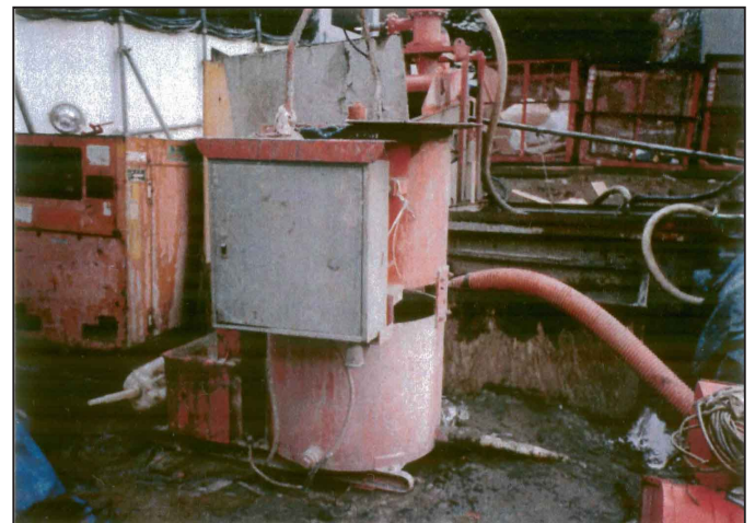
混練ミキサー
