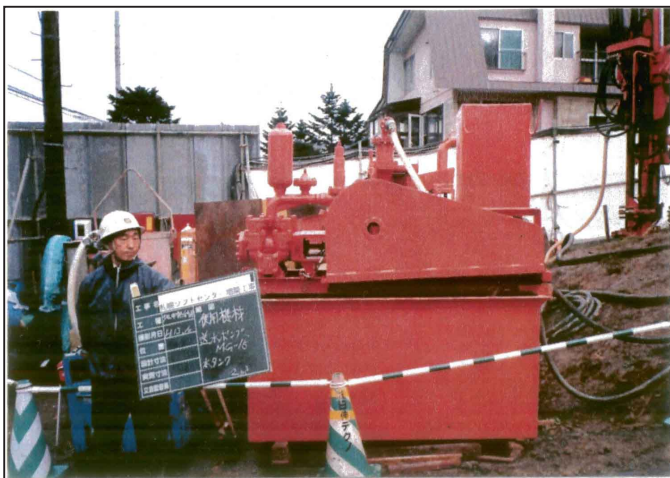
送水ポンプ MG-15 水タンク2m 3
